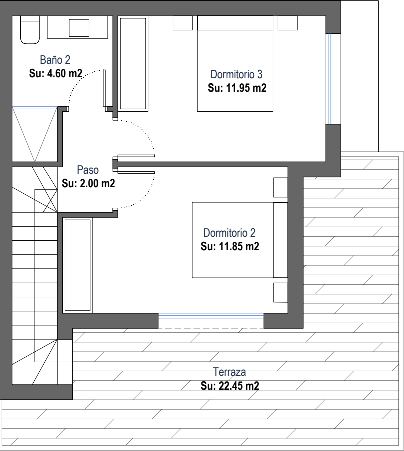
Planta Primera
