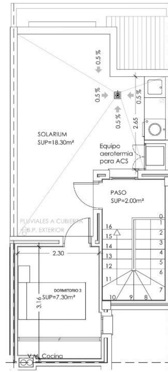
PLANTA TRASERO
