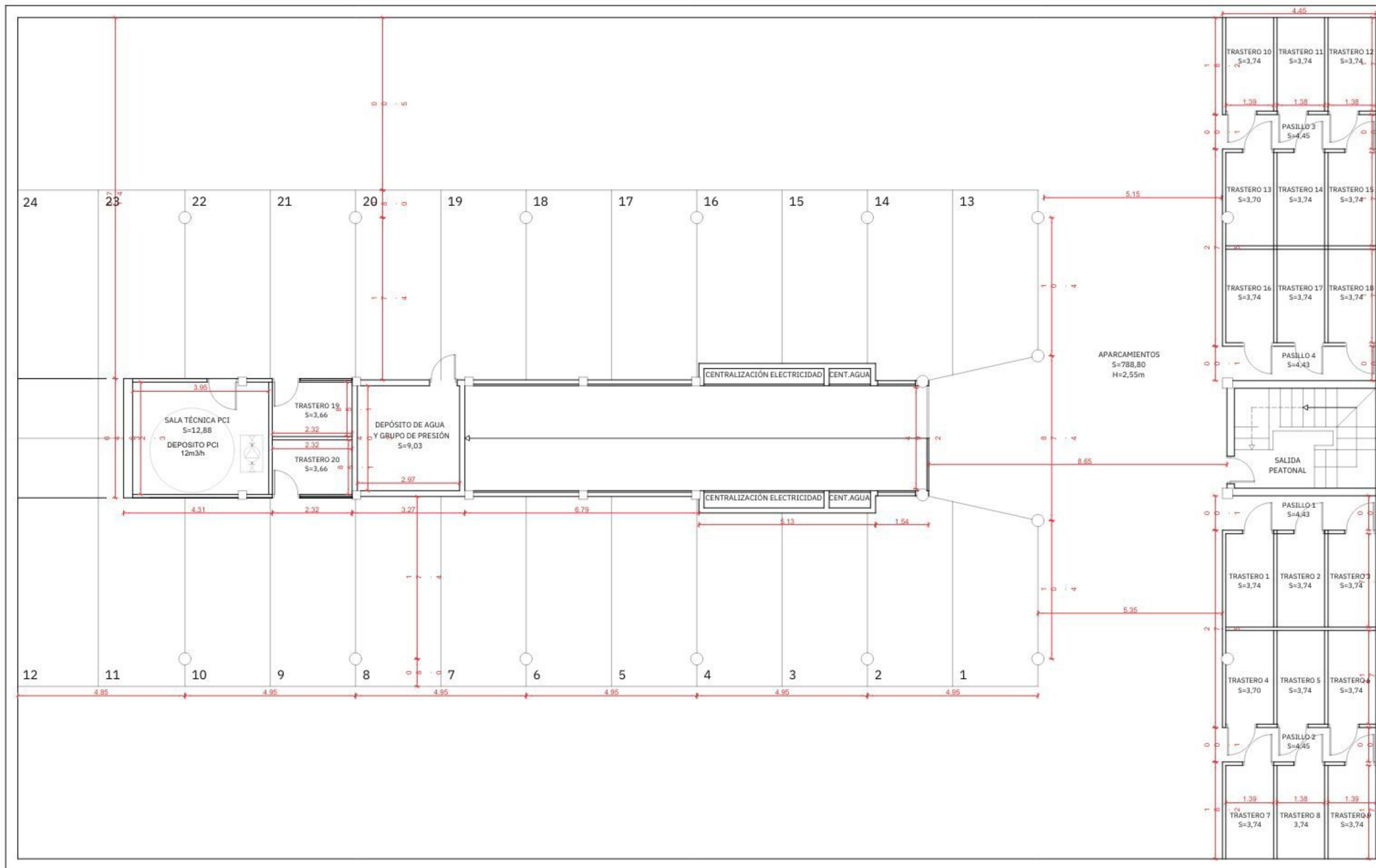
PLANTA GARAJE
