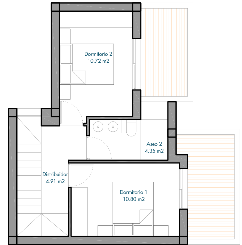
PLANTA PRIMERA
