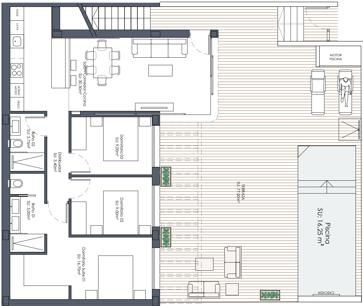
PLANTA BAJA
