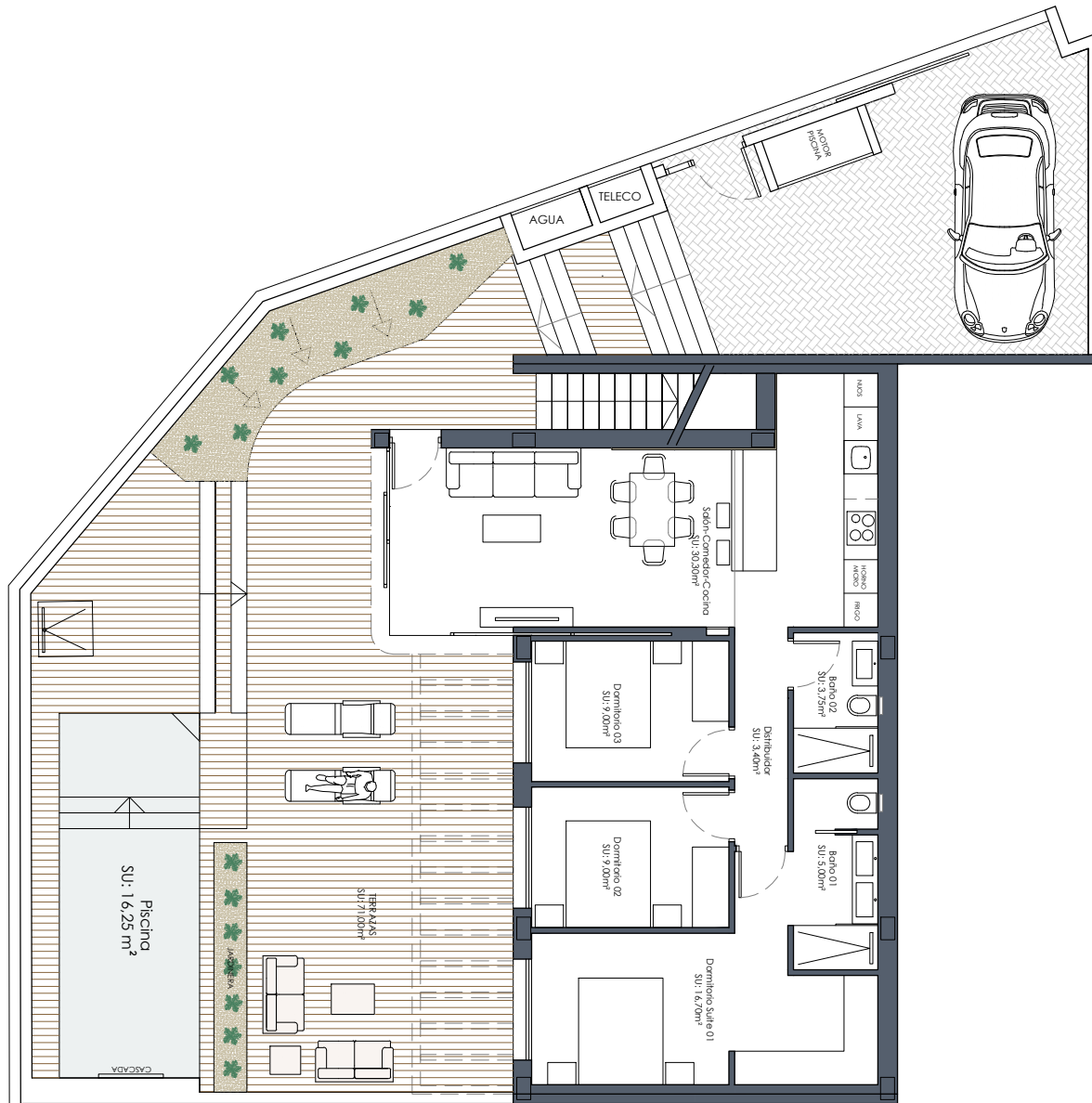
PLANTA BAJA
